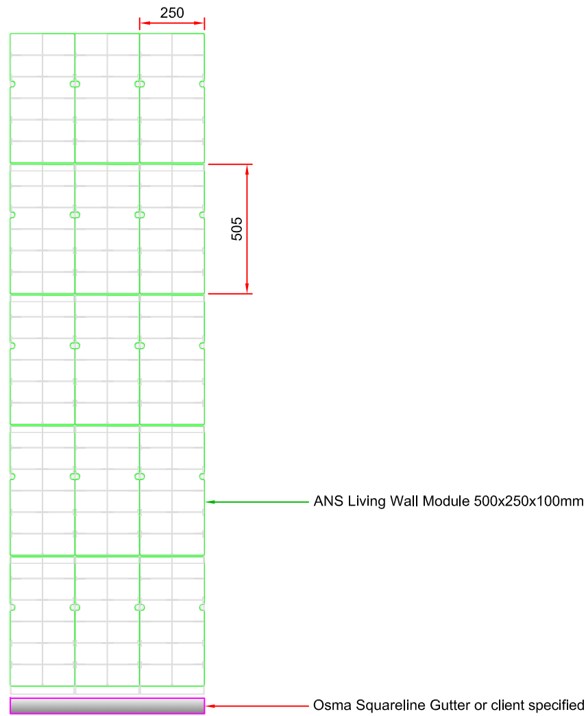
Front View Scale: 1:20
